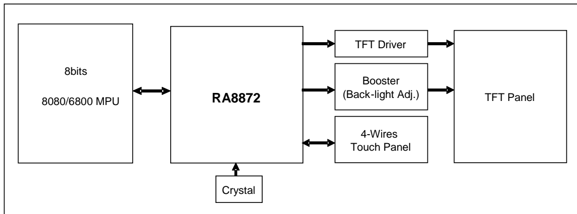
图 3-2：系统方块图
