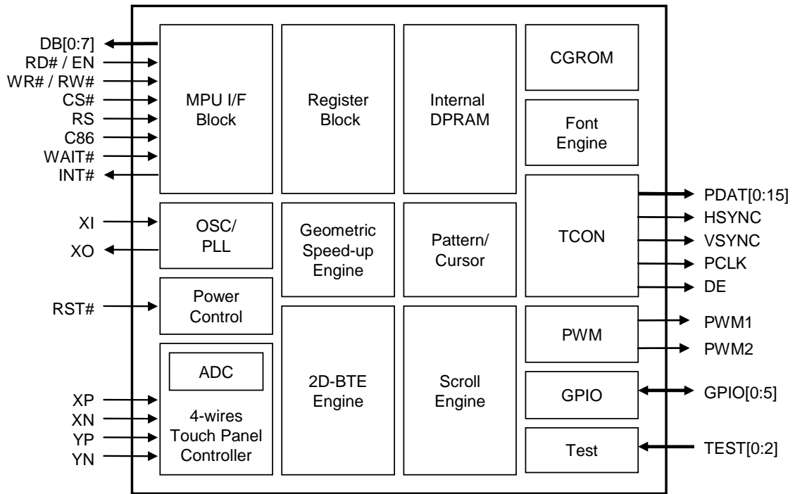
图 3-1：内部方块图
