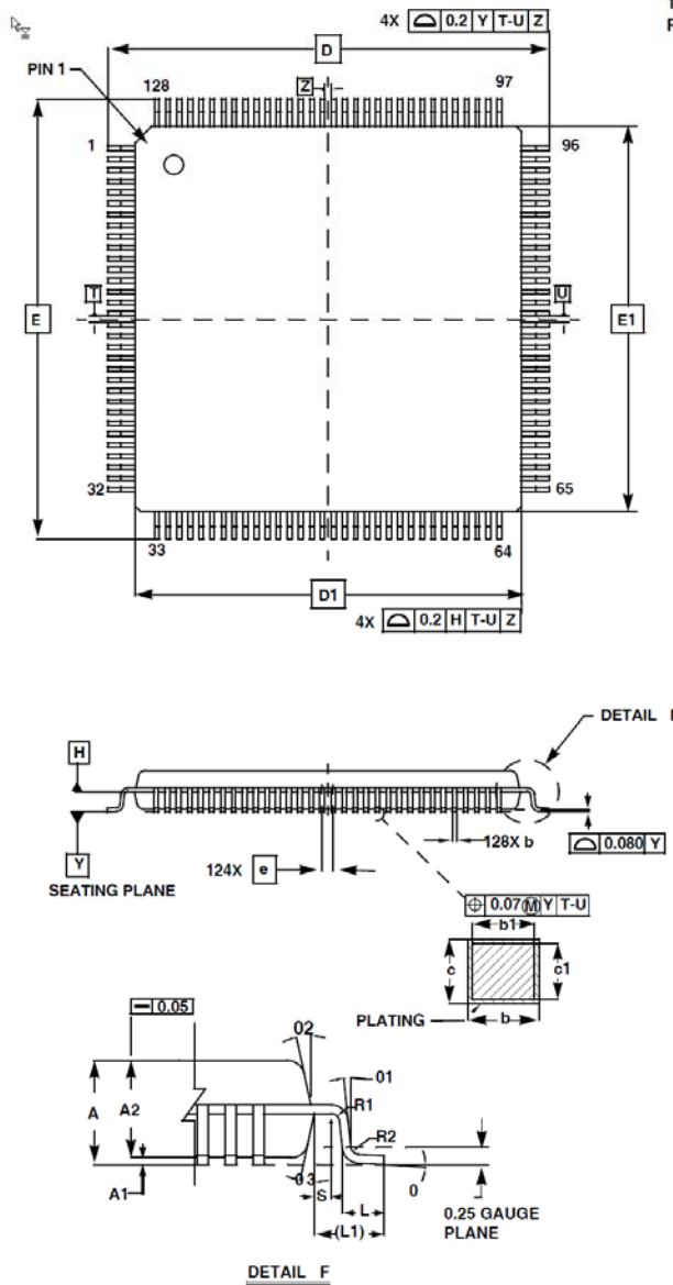
圖 3-2 : RA8871 Package Outline Dimensions
