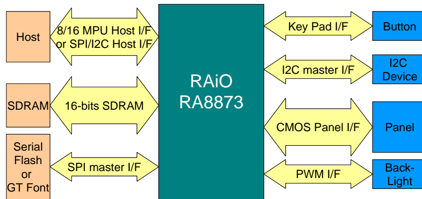
圖 1-1 : System Diagram
