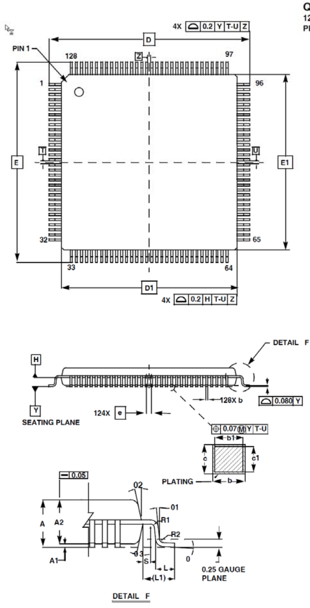
圖 3-2 : RA8873 Package Outline Dimensions
