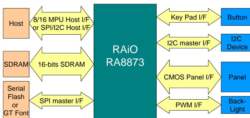
圖 1-1 : System Diagram
