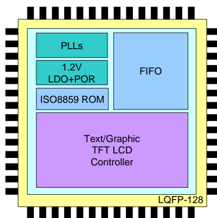
圖 1-2 : Chip Diagram
