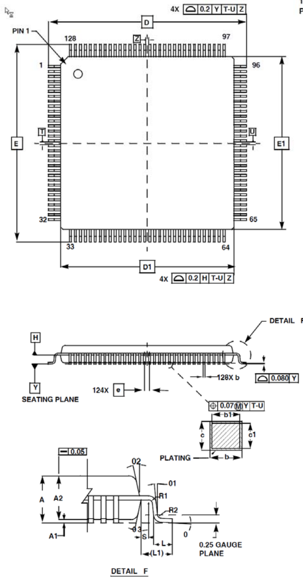
圖 3-2 : RA8873 Package Outline Dimensions
