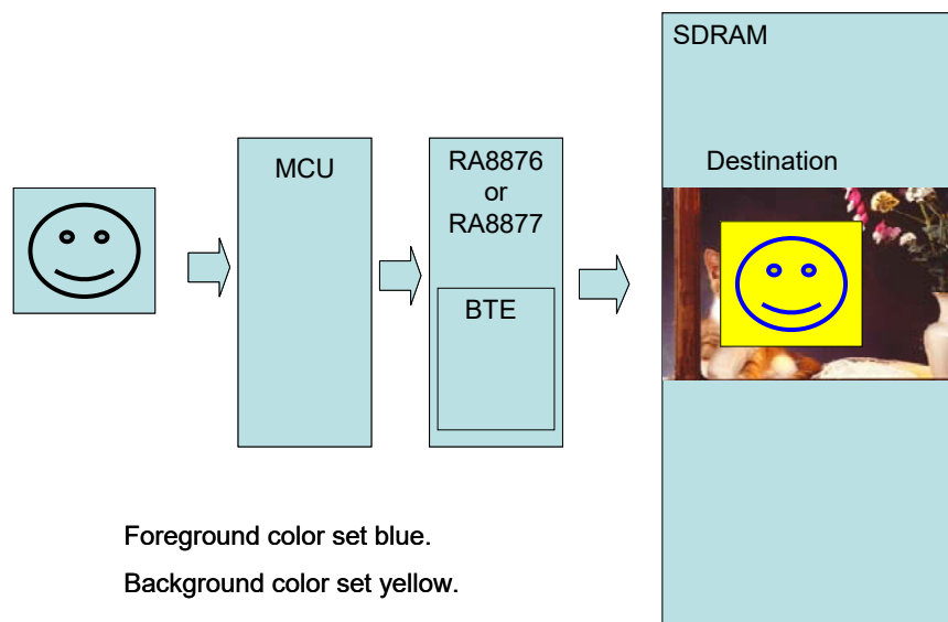
图 4-36：硬體資料流程
