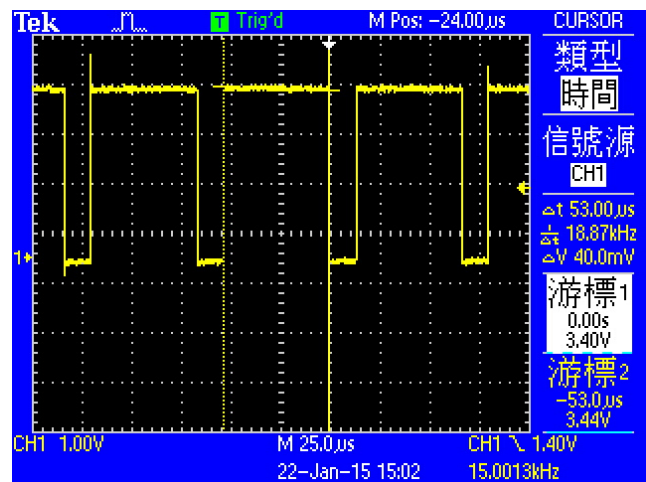
图 7-5 : PWM1 輸出高电位的时间
