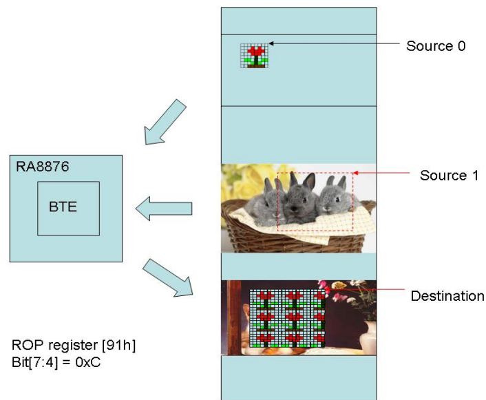
图 4-72：硬體資料流程
