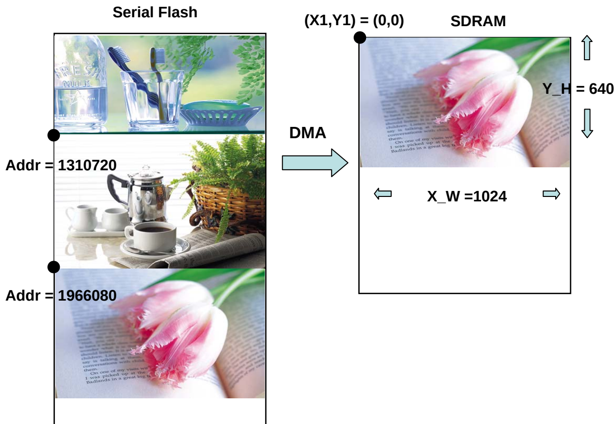
圖 3.4: 使用 DMA 功能將串列式 Flash 中的資料寫到 SDRAM 中
