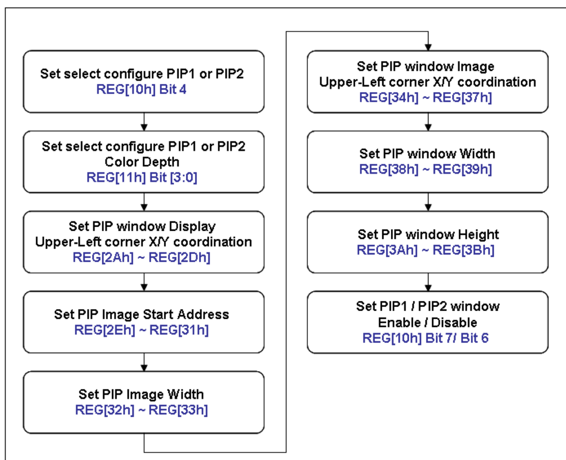
圖 5-1：流程圖
