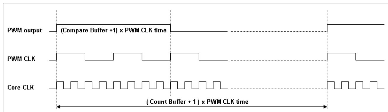
圖 7-1：PWM 時序圖
