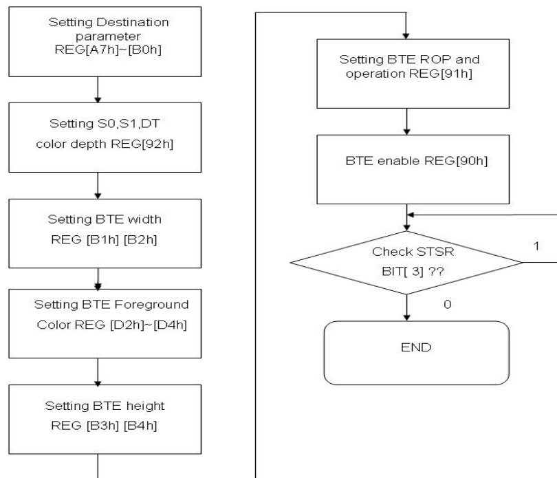
圖 4-3 : 流程圖
