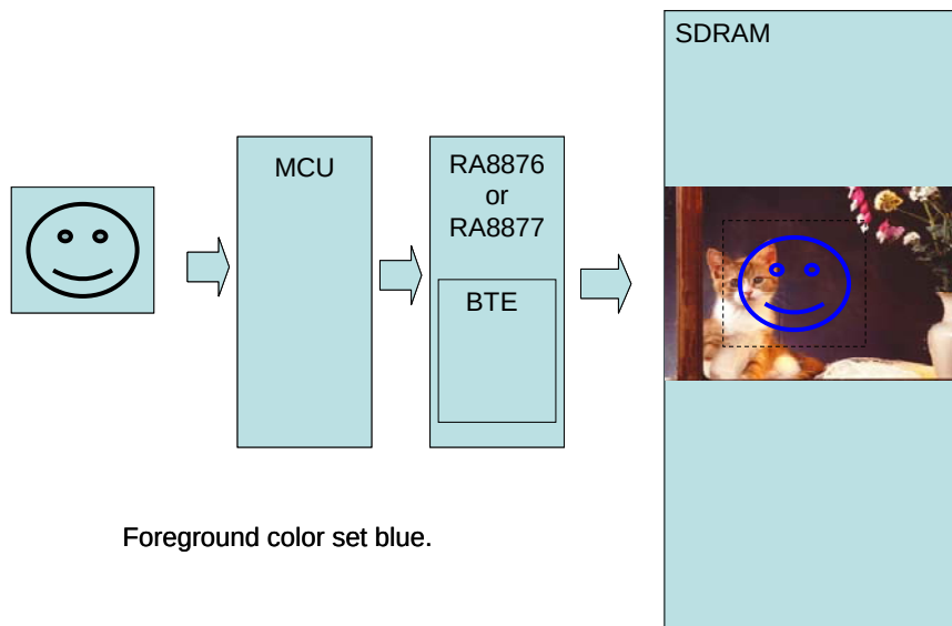
圖 4-44：硬體資料流程
