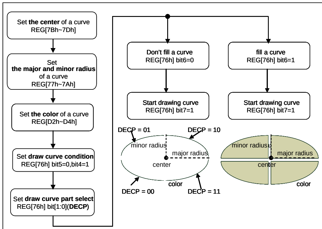
圖 2-4 畫圓弧與圓弧形填滿的程式流程圖
